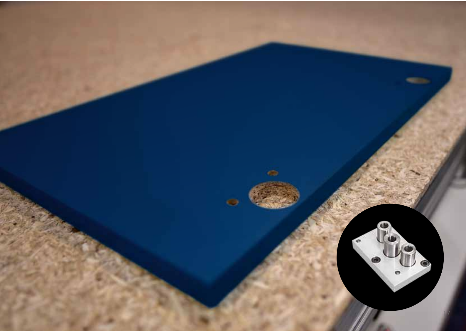
SCHARNIERBOHRUNG: DREI ARBEITSSCHRITTE IN EINEM! Drei Bohrungen können gleichzeitig ausgeführt werden mit einem einzigen integrierten Bohrkopf.
