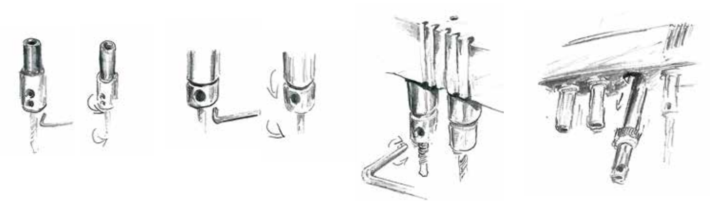
RO.AX SPINDEL Keinerlei Spiel mehr während der Bearbeitung durch die neue RO.AX Technik (Rotoaxial spindle technology), die leistungsstärksten Bohrspindeln auf dem Markt mit einer Drehzahl von bis zu 8000 U/min.
