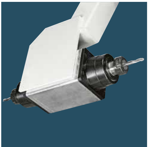
Herstellung von Türen und weiterer horizontaler Bearbeitungen, mit hohem Spanabtrag (Nuten, Scharnierfräsungen oder Schloßkasten) auf genaue und schnelle Art und Weise mit Elektrospindel mit zwei horizontalen Ausgängen.
